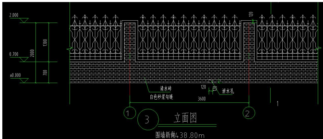
砖围墙成品铸铁栏杆示意图
