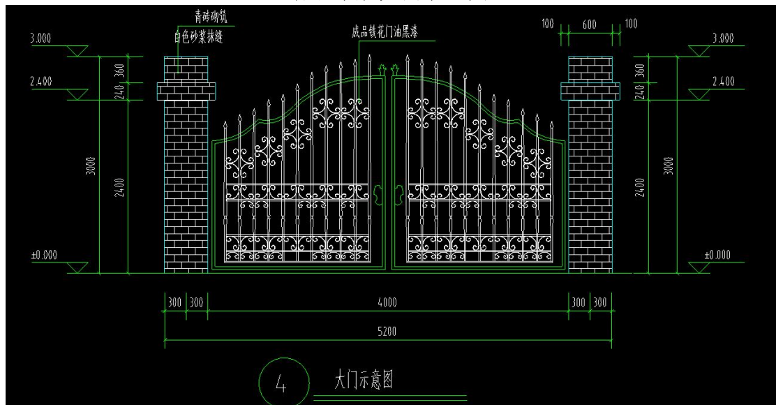
成品铁花大门示意图
